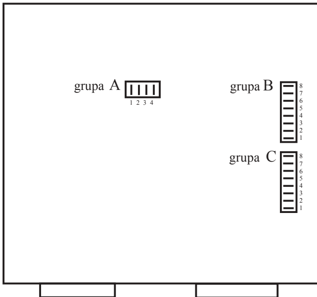
Rys. Układ zwor na płycie głównej centrali.
