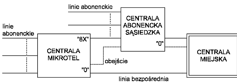
Rys. 1. Przykładowe rozwiązanie obejścia w centrali
