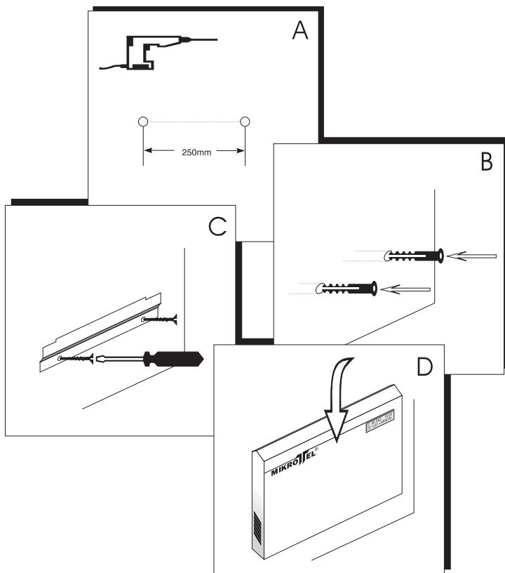
RYS.3. Montaż łącznicy.
