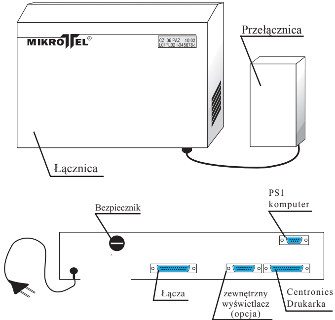
RYS.2. Wygląd zewnętrzny łącznicy i przełącznicy.
