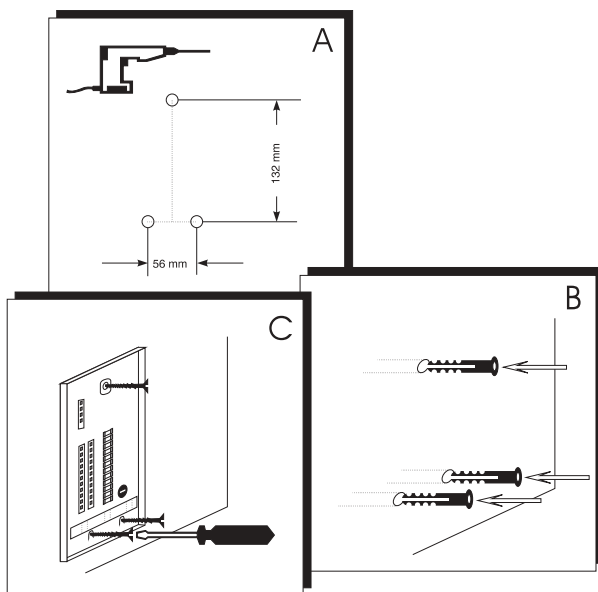
RYS.4. Montaż przełącznicy.
