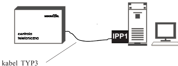
Rys.4. Sposób podłączenia w przypadku dużej odległości komputera od centrali (10 - 100 m).
