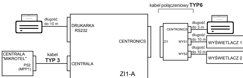
Rys. 5. Schematyczna prezentacja możliwości wykorzystania zdalnego interfejsu ZII-A przy pracy z wyświetlaczami i drukarkami.
